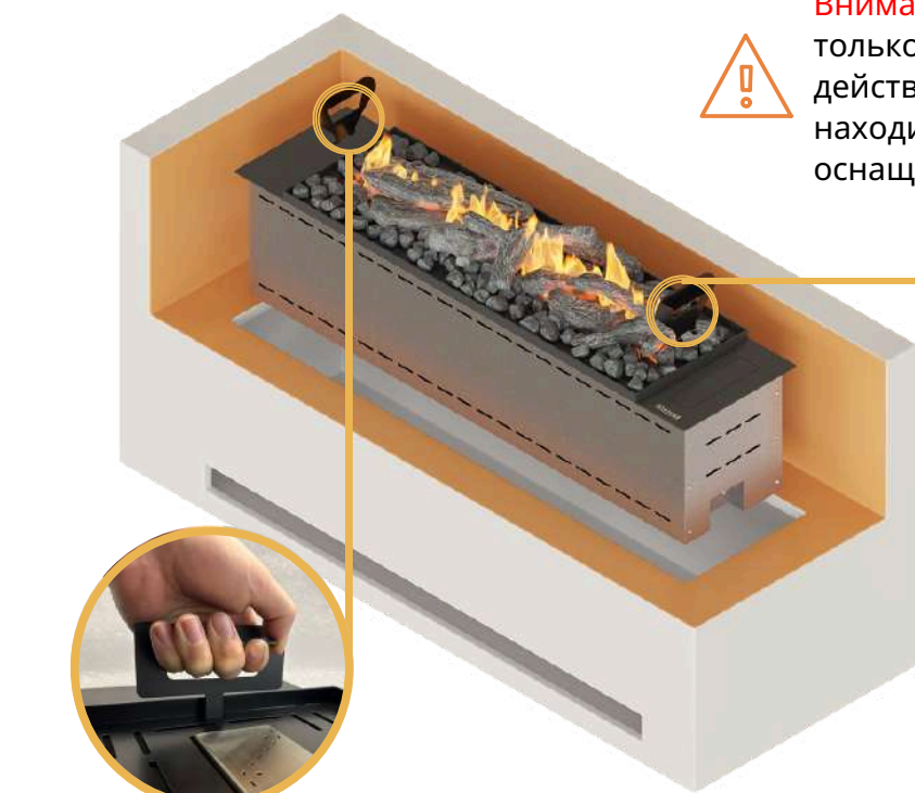
Монтажные держатели
