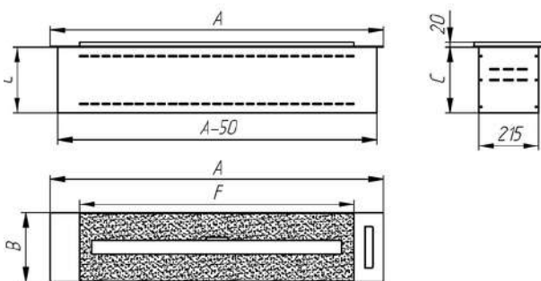
Габаритные размеры автоматической топки Prime
