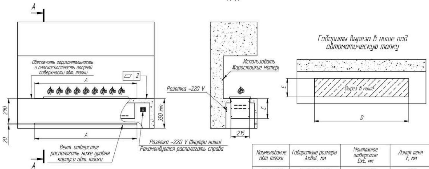
Габаритные размеры автоматической топки Prime
